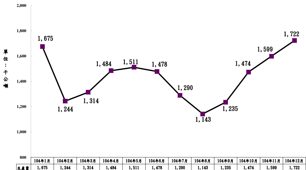
圖 5-4-1 104 年 1 月至 12 月南部地區砂石成品生產走勢
