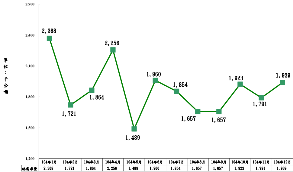
圖 4-7-1 104 年 1 月至 12 月中部地區砂石成品需求走勢
