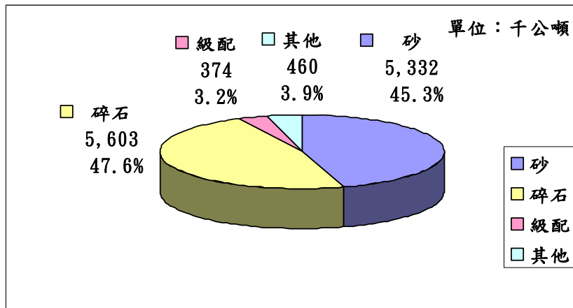
圖 3-4-2 104 年北部地區砂石成品生產結構
