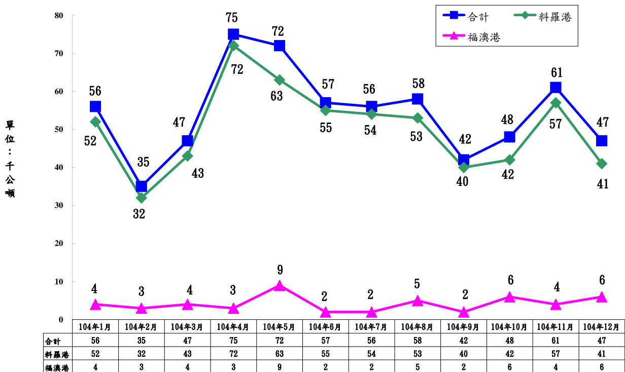
圖 7-2-1 104 年 1 月至 12 月金馬地區進口砂石量走勢
