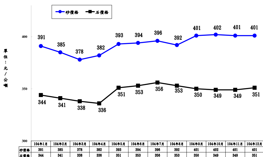
圖 4-9-1 104 年 1 月至 12 月中部地區自產砂石成品價格走勢
