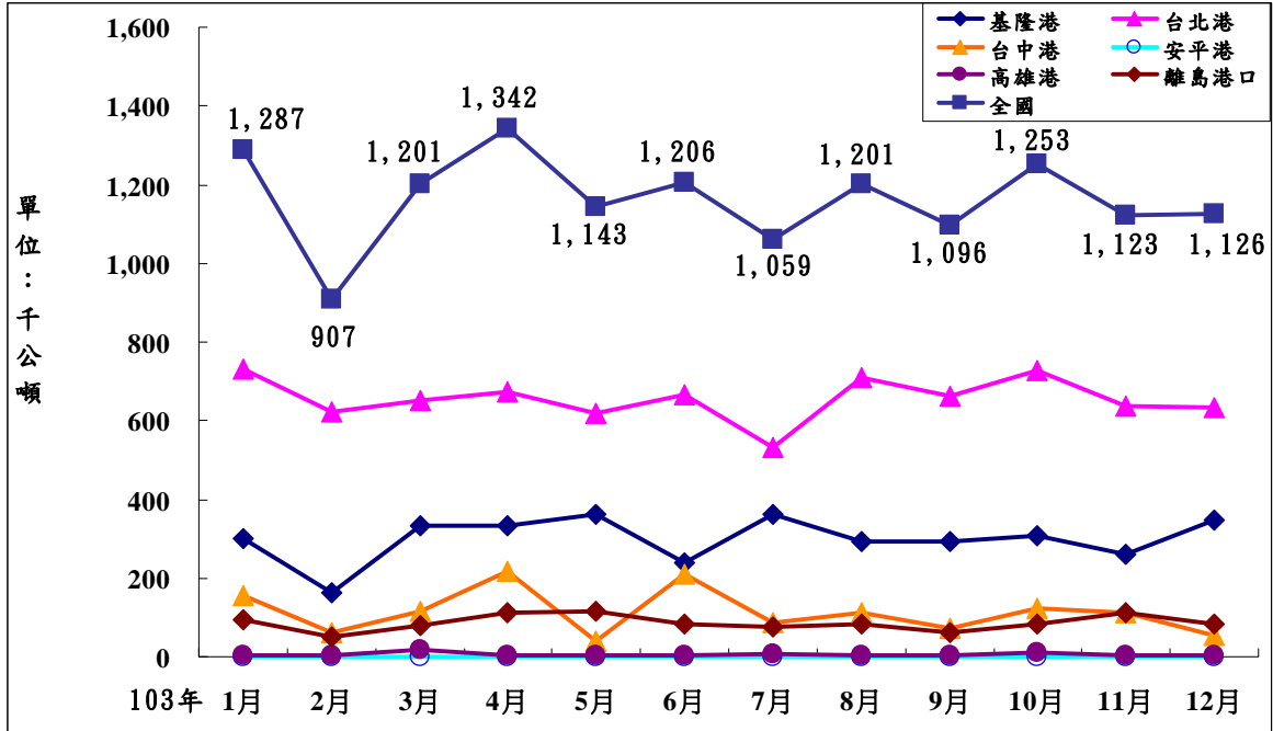
圖 2-10-3 104 年 1 月至 12 月臺灣全區各港口進口砂石量走勢
