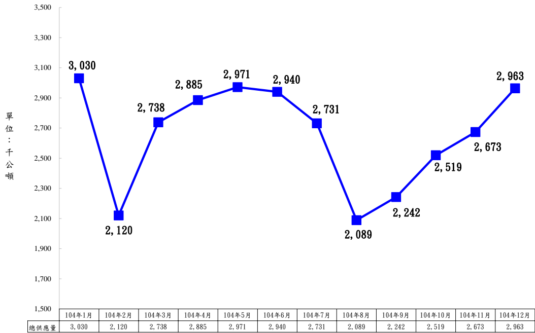
圖 5-6-1 104 年 1 月至 12 月南部地區砂石成品供應走勢
