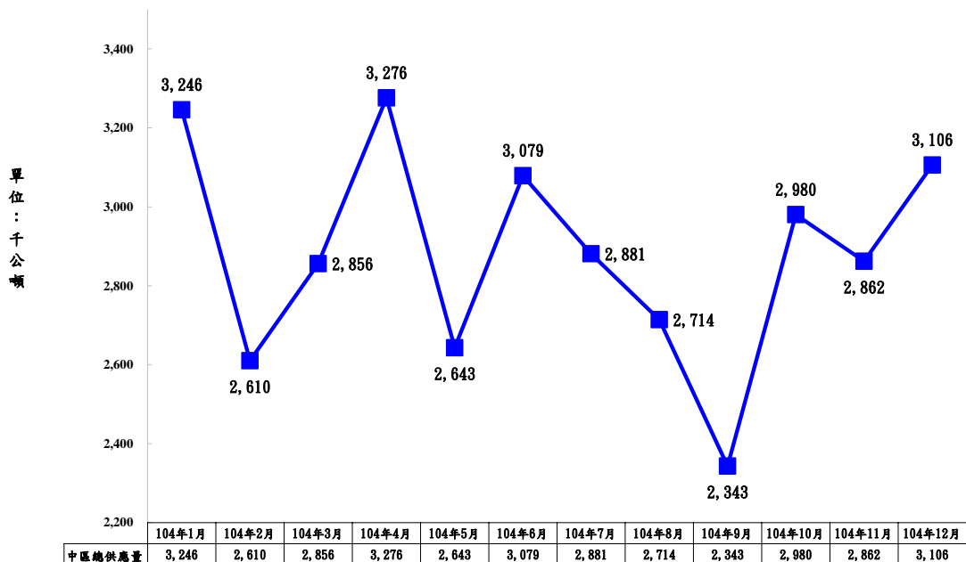
圖 4-6-1 104 年 1 月至 12 月中部地區砂石成品供應走勢
