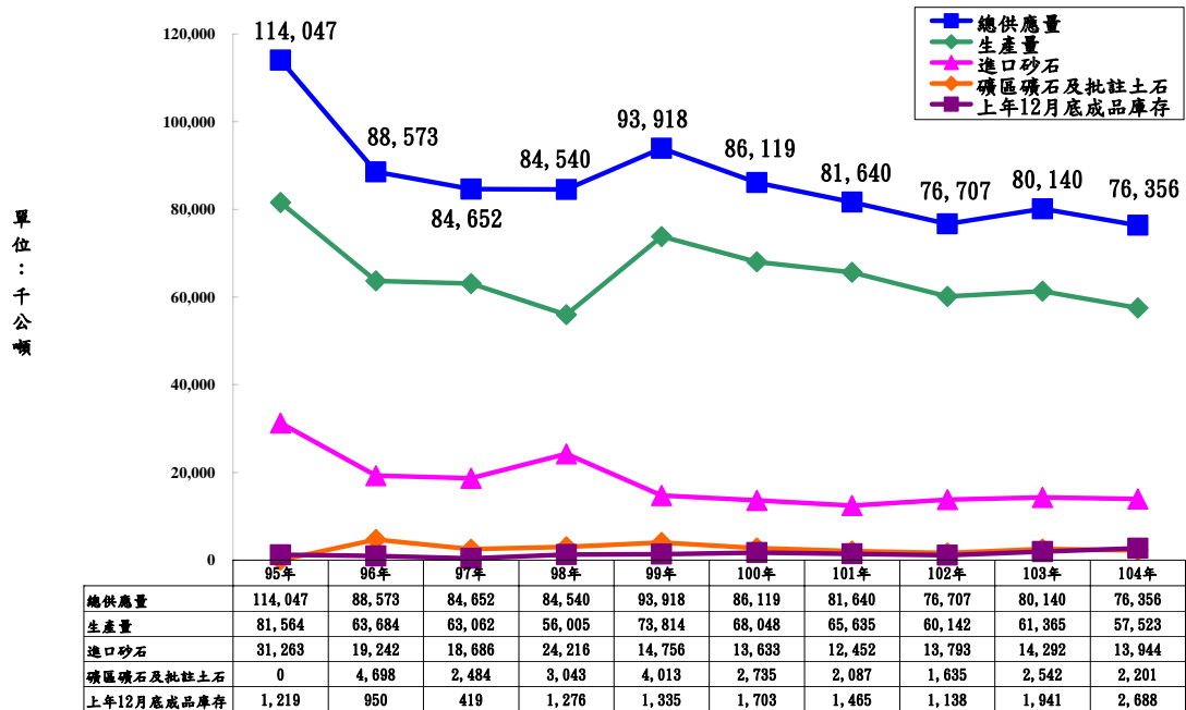
圖 2-6-1 95 年至 104 年臺灣全區砂石成品供應走勢
