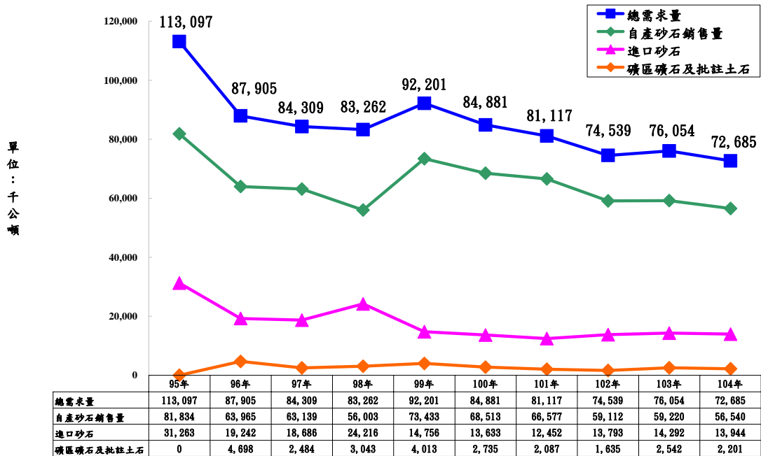
圖 2-7-1 95 年至 104 年臺灣全區砂石成品需求走勢
