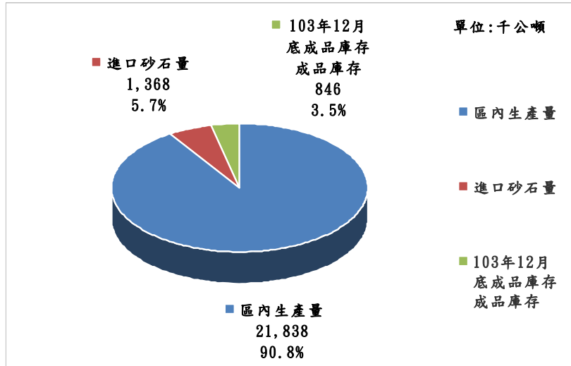
圖 4-6-2 104 年中部地區砂石成品供應結構
