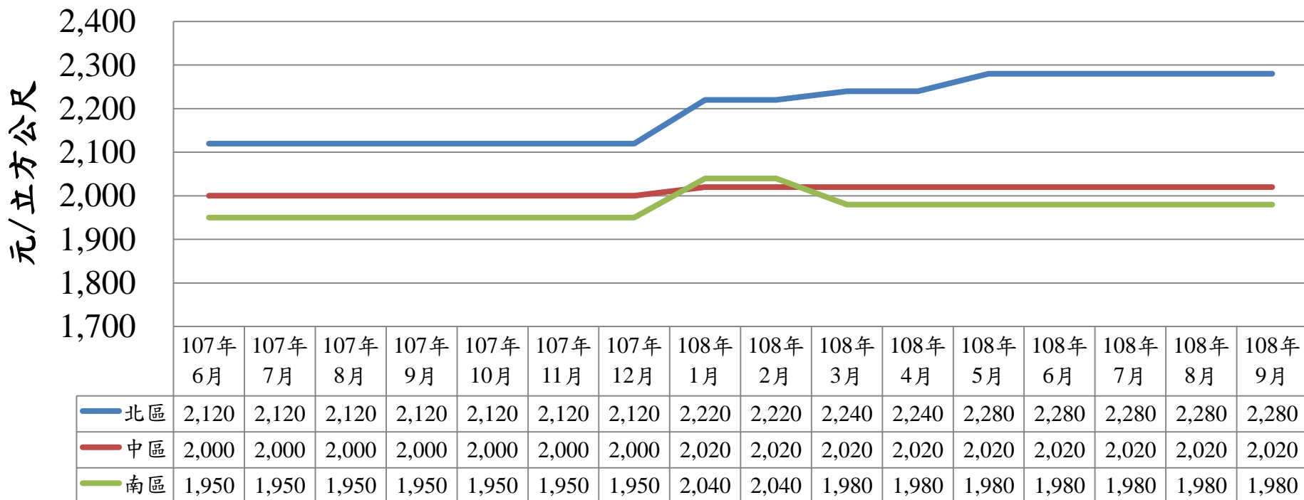
107年6月至108年9月北中南區預拌混凝土價格表
