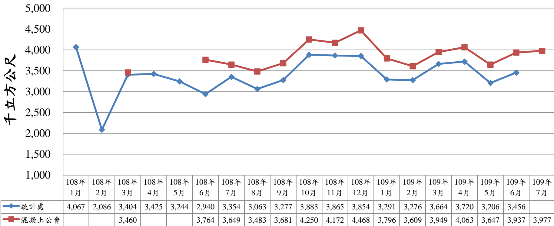
108年至109年6月預拌混凝土產量統計表
