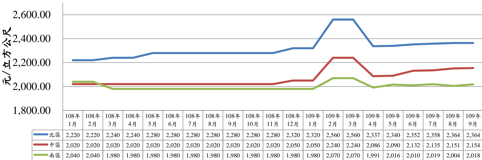
108年至109年9月北中南區預拌混凝土價格表
