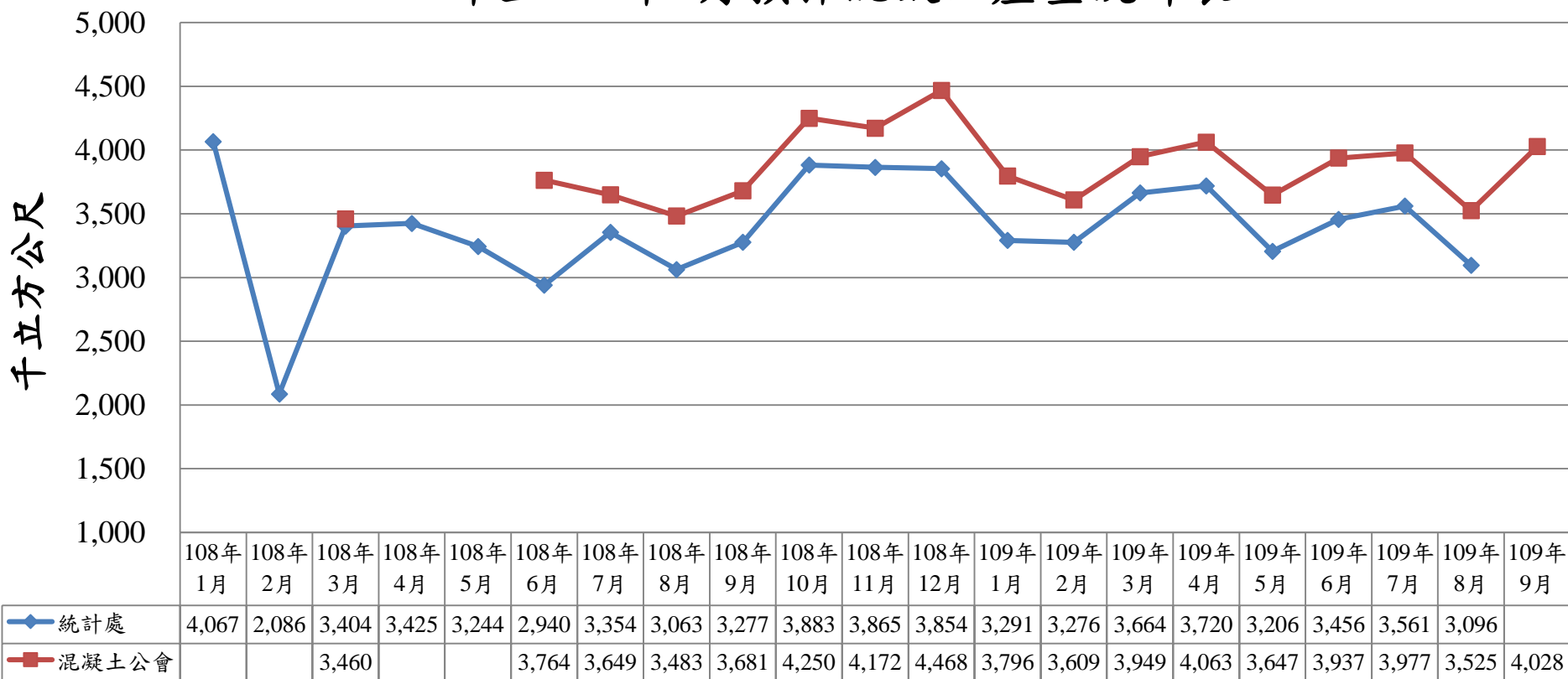
108年至109年9月預拌混凝土產量統計表
