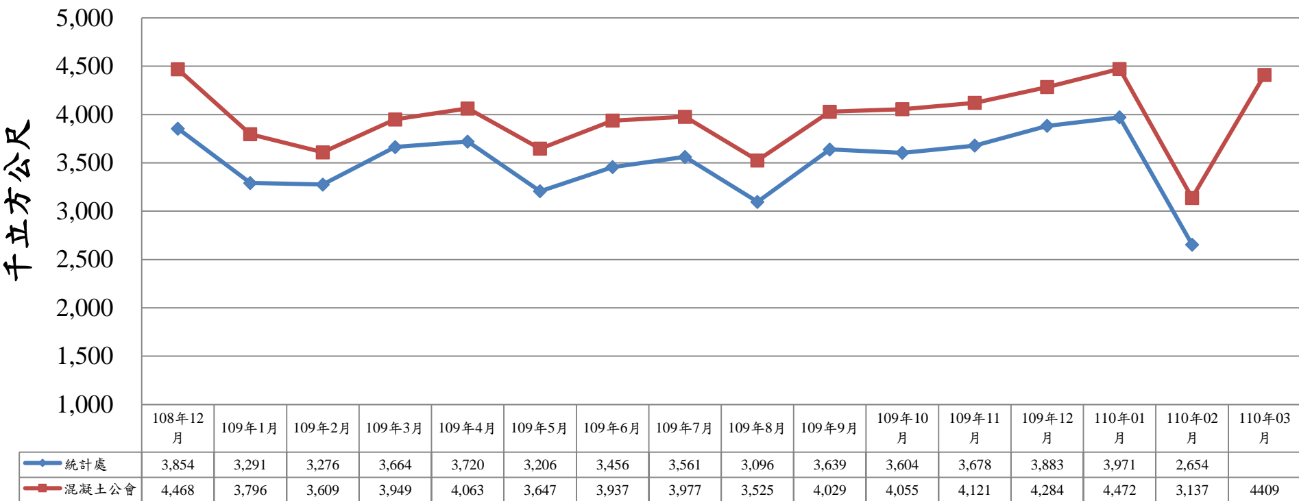
108年12月至110年3月預拌混凝土產量統計表
