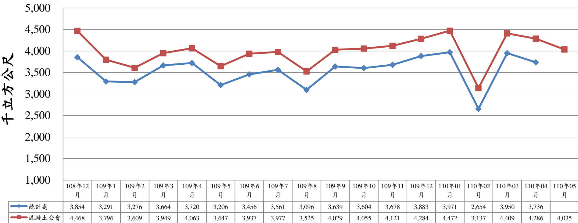
108年12月至110年5月預拌混凝土產量統計表
