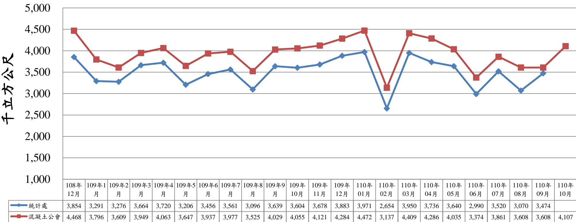
108年12月至110年10月預拌混凝土產量統計表
