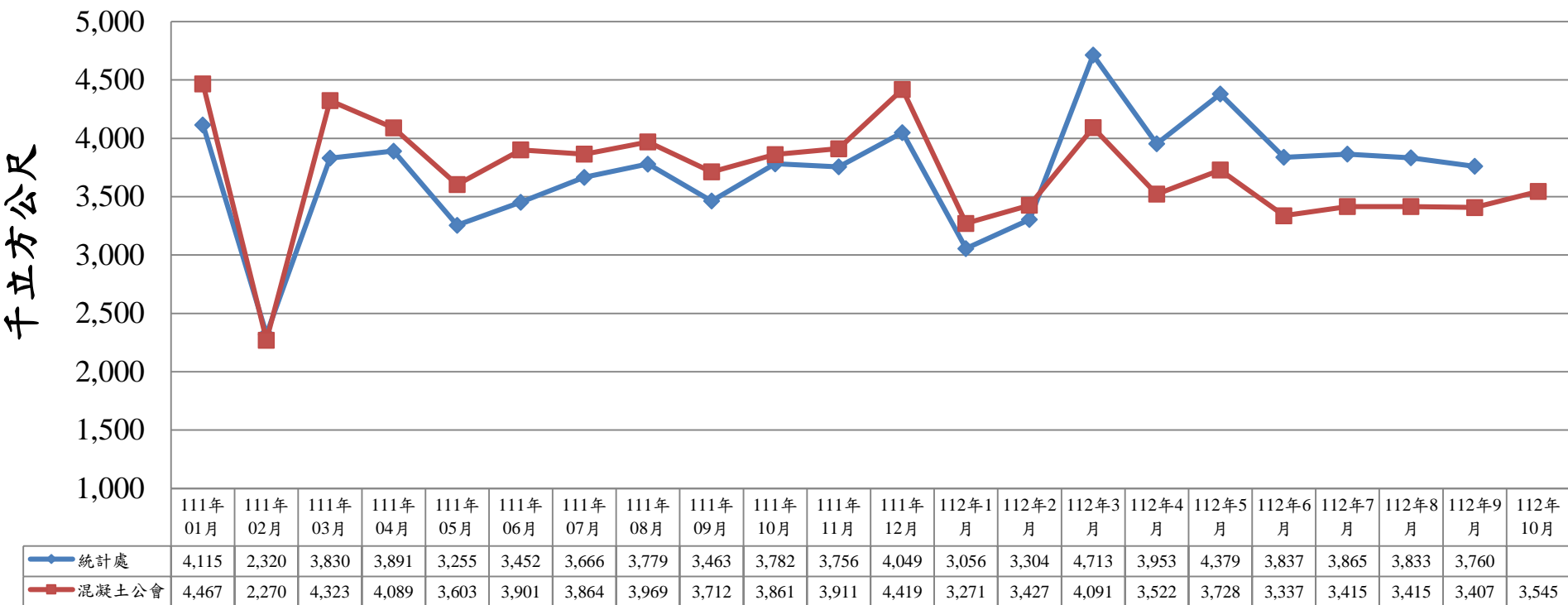
111年1月至112年10月預拌混凝土產量統計表
