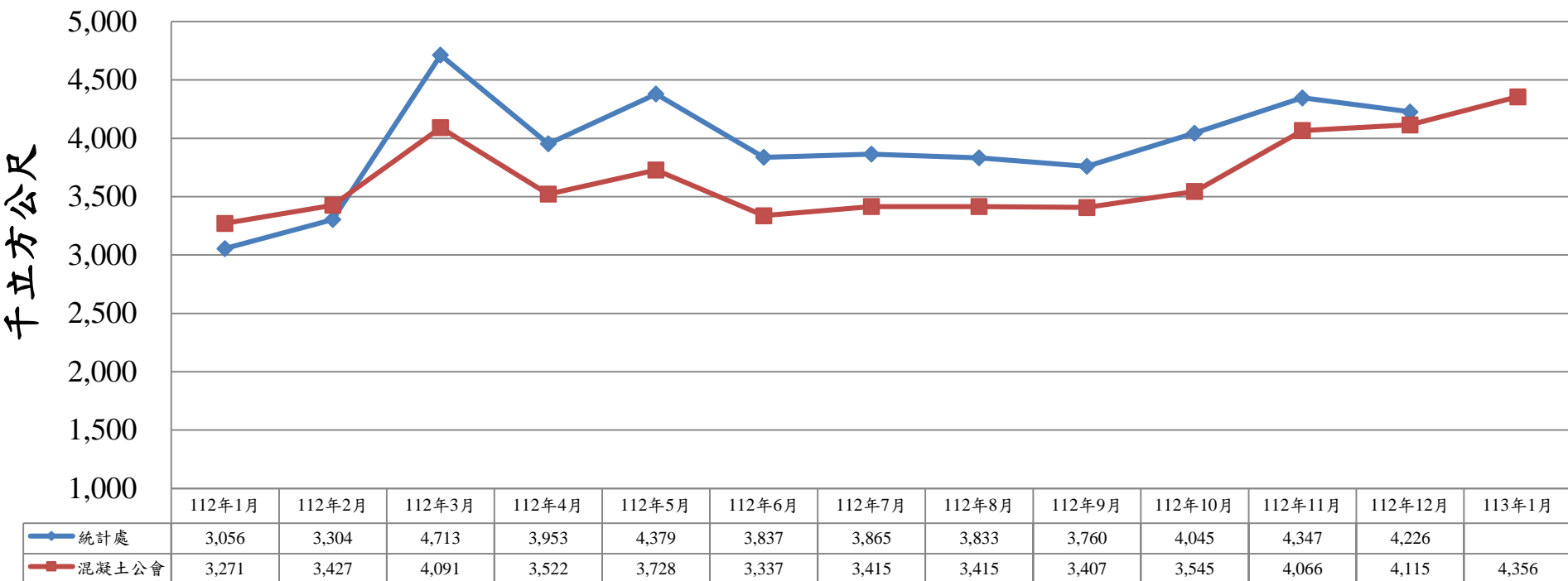
112年1月至113年1月預拌混凝土產量統計表
